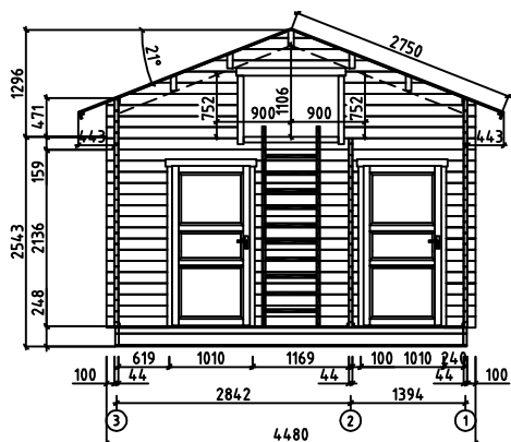
Wall- Seinä-Vägg B
