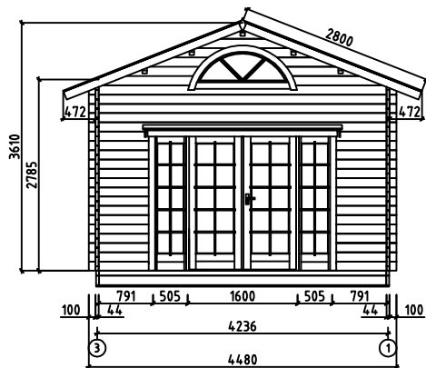
Wall- Seinä-Vägg A
